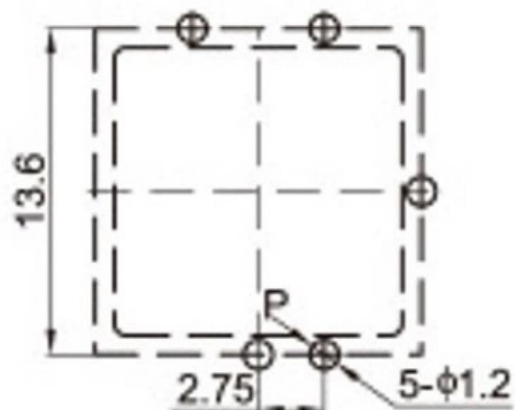
印制线路板 P.C.B
